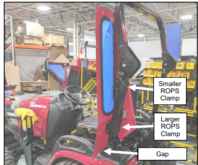
Fig. 3.2 (Install Left Rear Leg)
