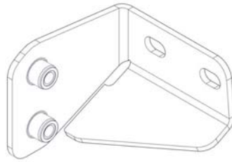
ROPS CLAMP BRKT P/N: 8SV-K6247-21
