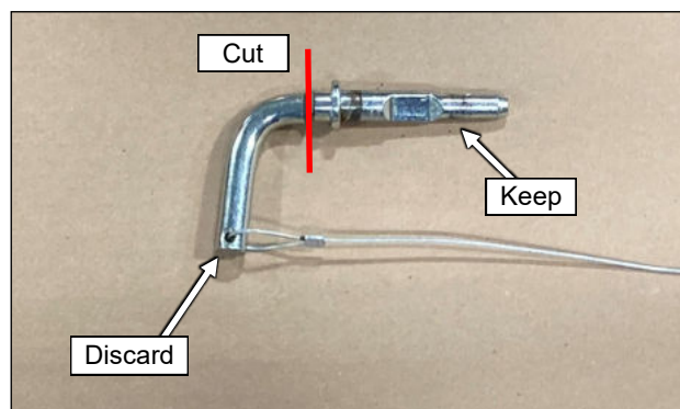
Fig. 3.6 (Trim ROPS pins)
