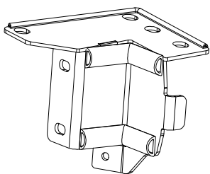
DYNAMO P/N: 9SV-9ALT-06
