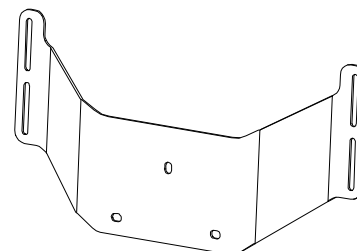
HEADREST MOUNT P/N: 8SV-SM-02378
